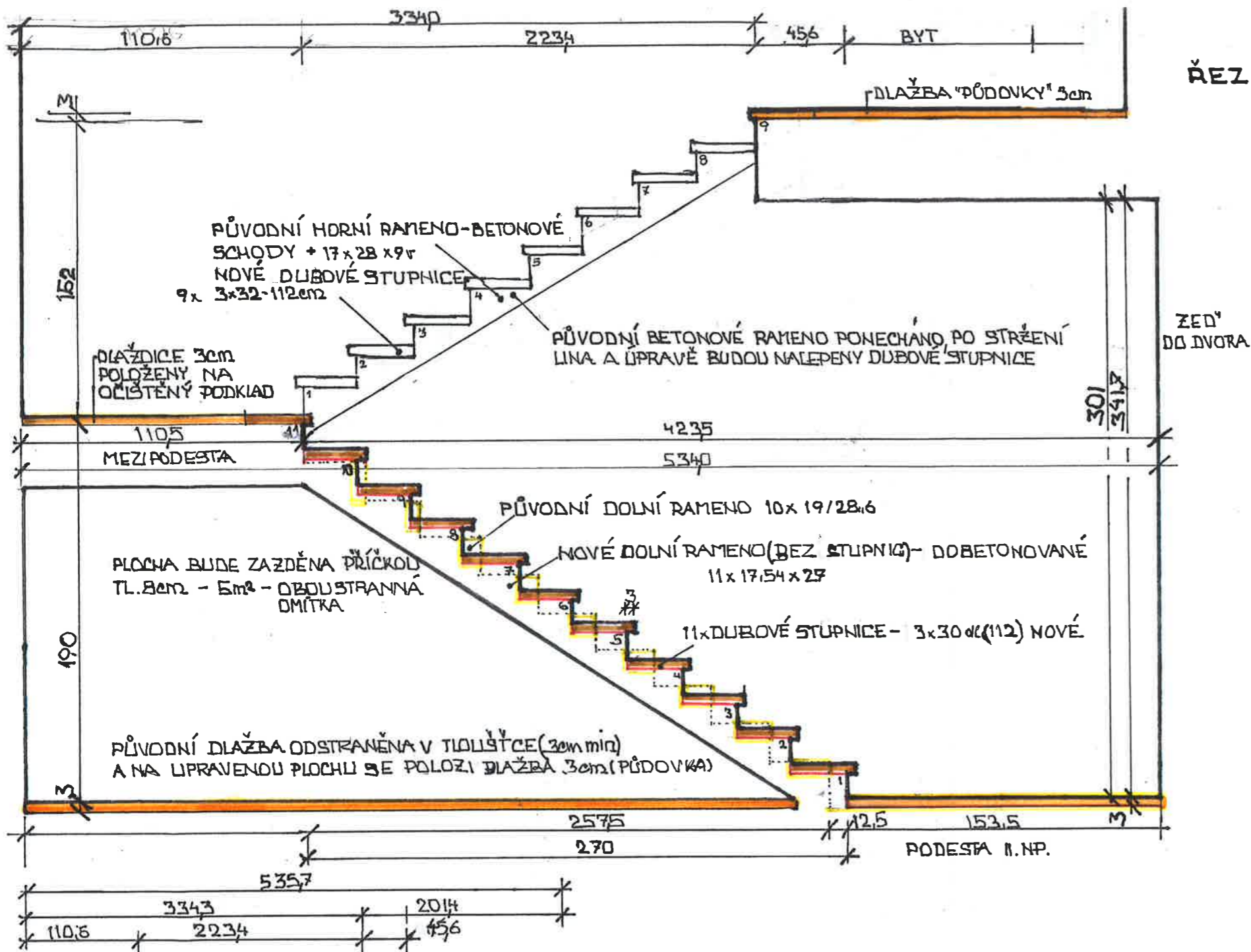
SCHÉMA III. PODLAŽÍ 1:50
