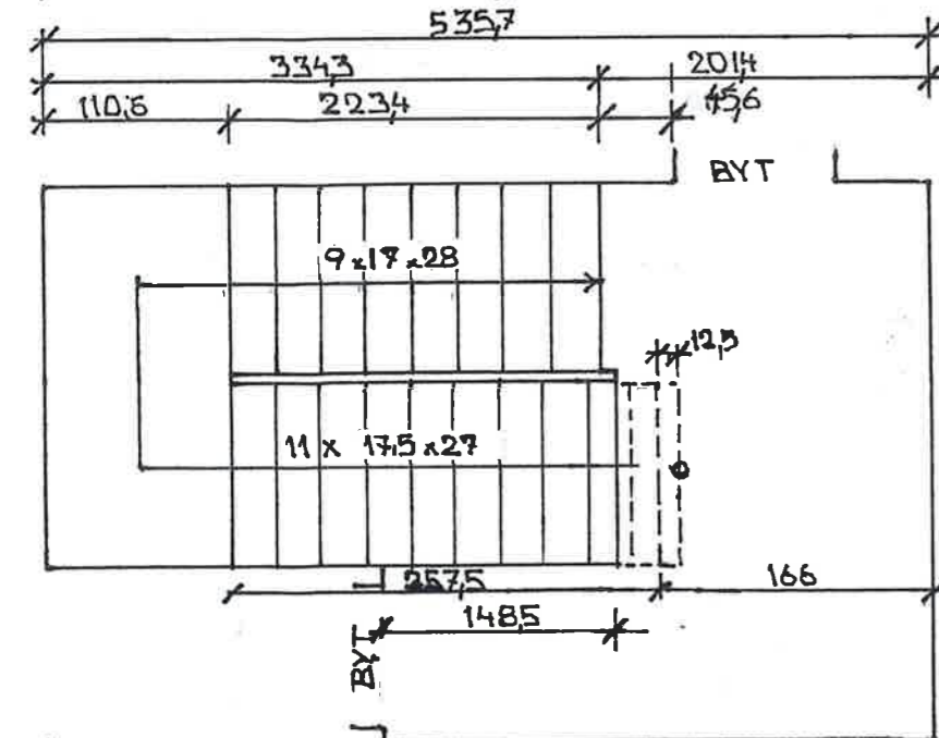
SCHÉMA III. PODLAŽÍ 1:50
